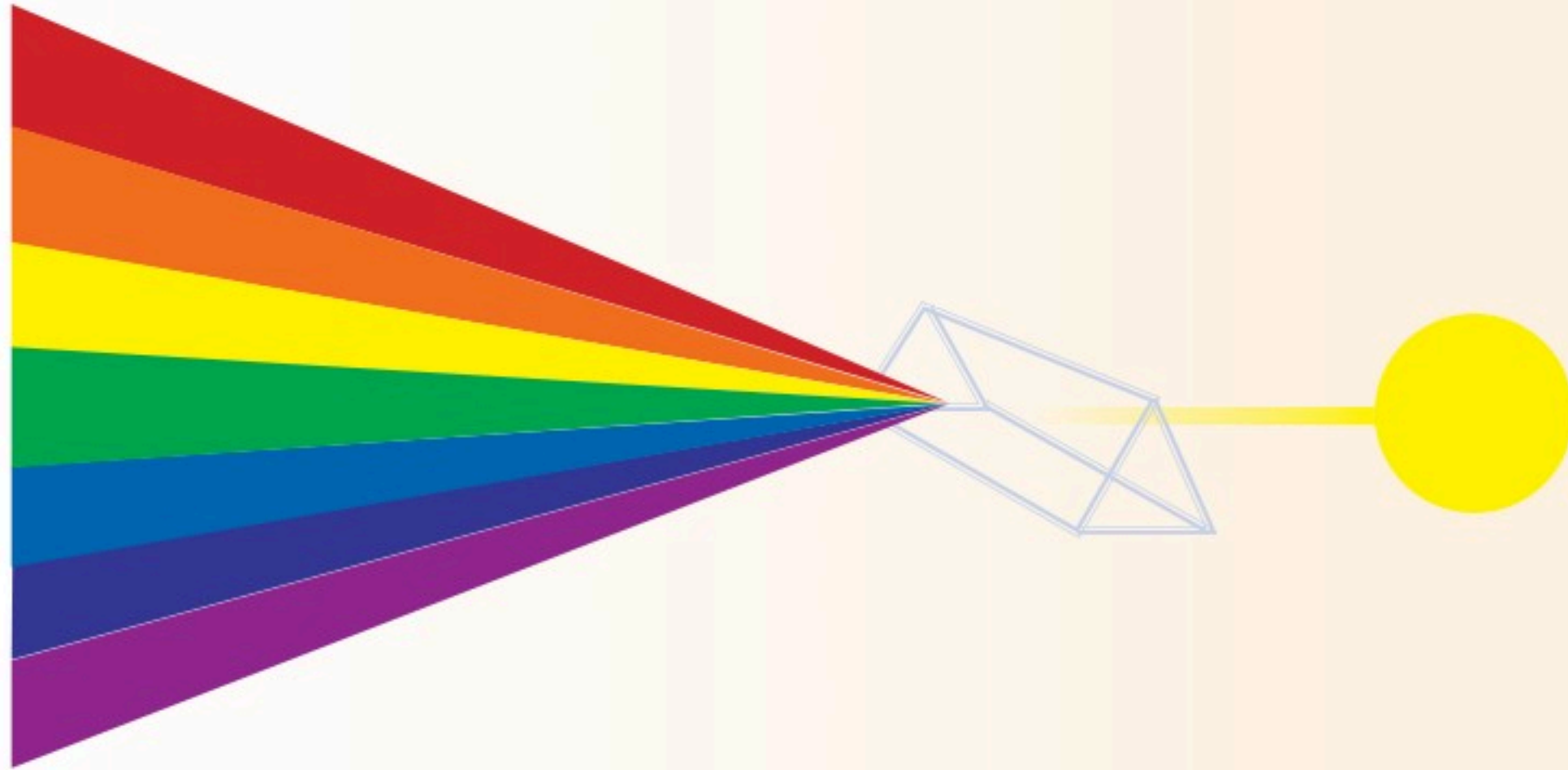
شكل (٥٨): ظاهرة الانكسار وألوان الطيف.
